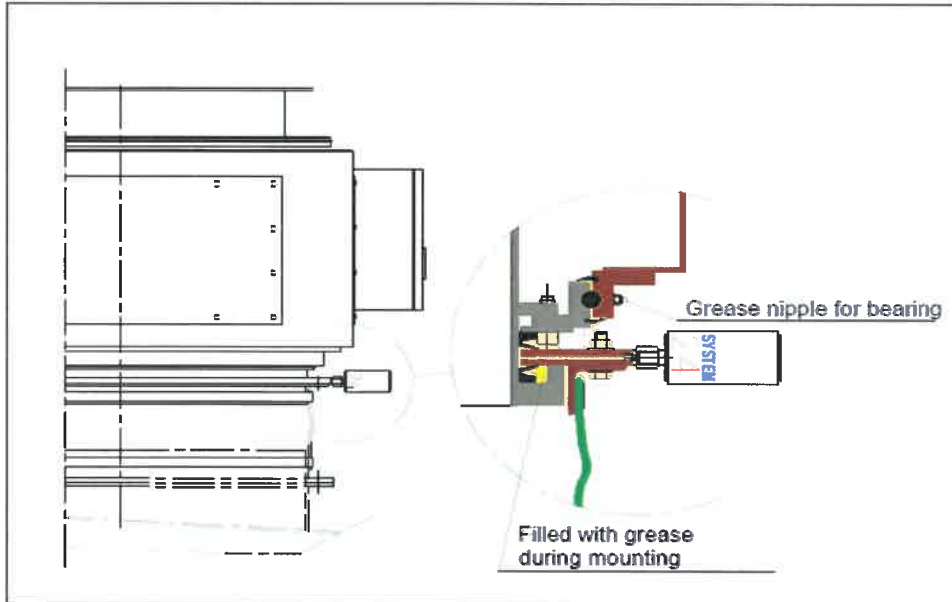
Rys. nr 6.13.20. Widok przekroju smarowania uszczelnienia pierścienia ślizgowego.
