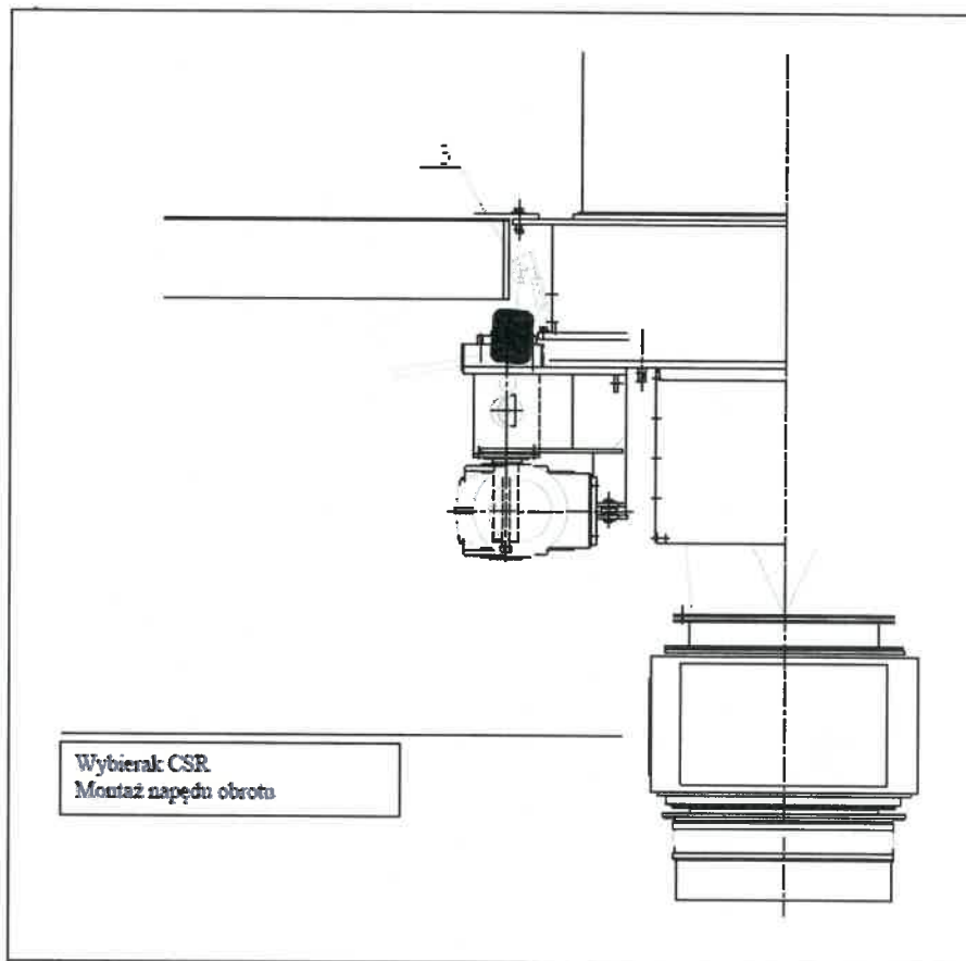
Rys. nr 6.13.26. Montaż napędu obrotu.
