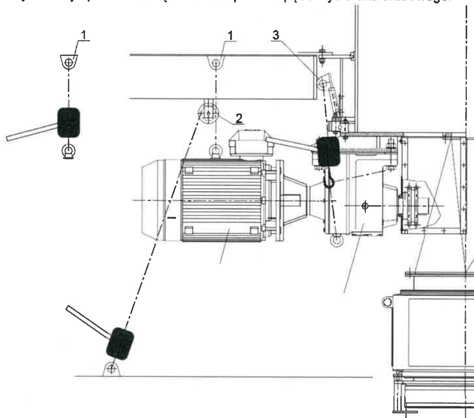
Rys. nr 6.13.25. Przykładowy sposób rozwiązania transportu napędu wybieraka śrubowego.
