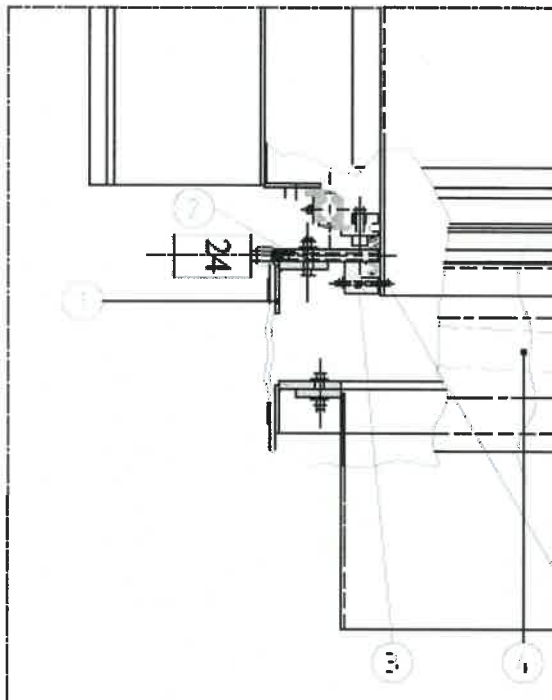
Rys. nr 6.13.24. Widok usytuowania uszczelki V rury odprowadzającej.
