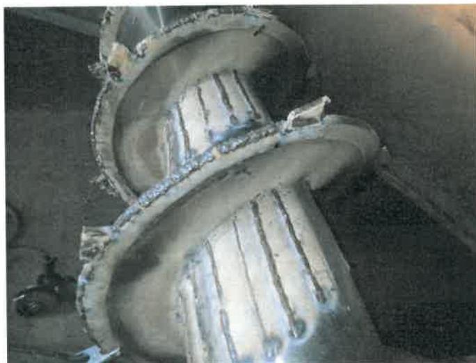
Rys. nr 6.13.17. Widok śruby wygarniacza w trakcie napawania śruby.
