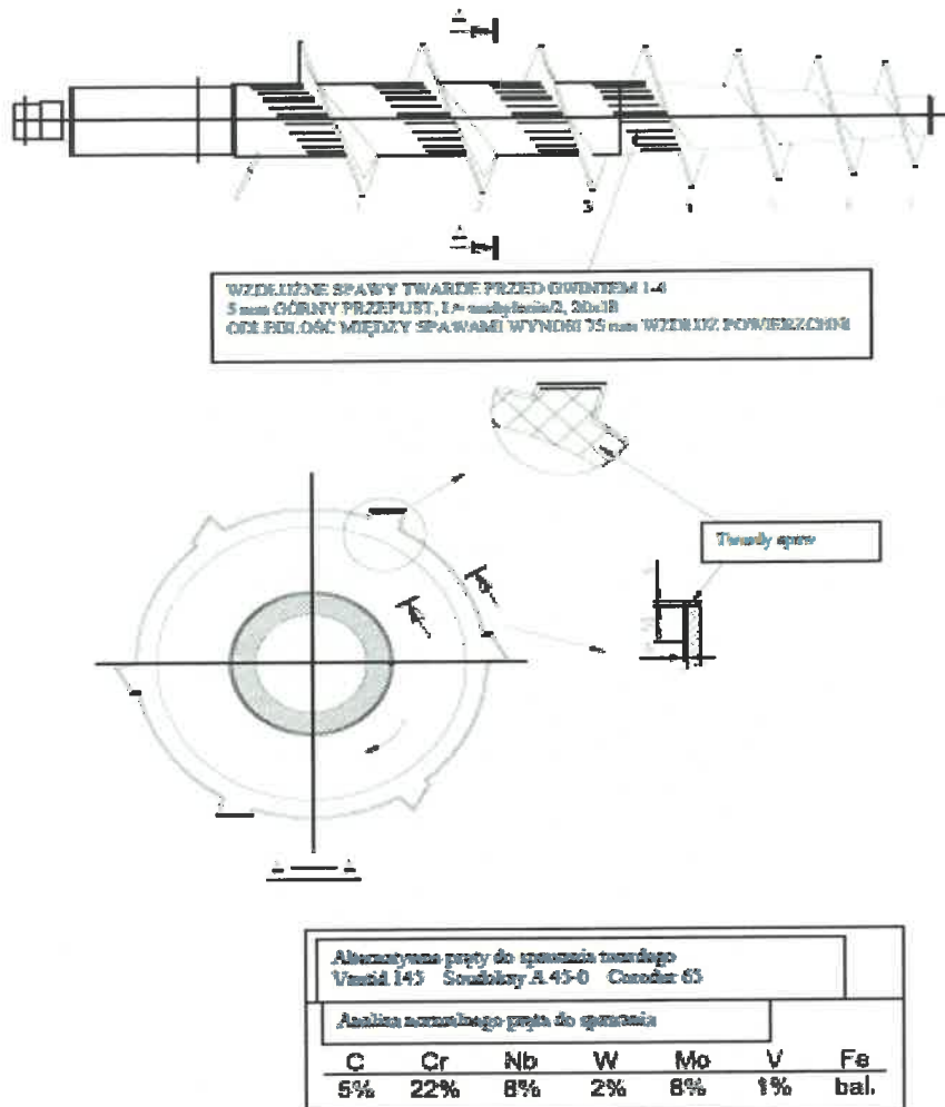
Rys. nr 6.13.16. Wytyczne producenta do napawania śruby wygarniacza.
