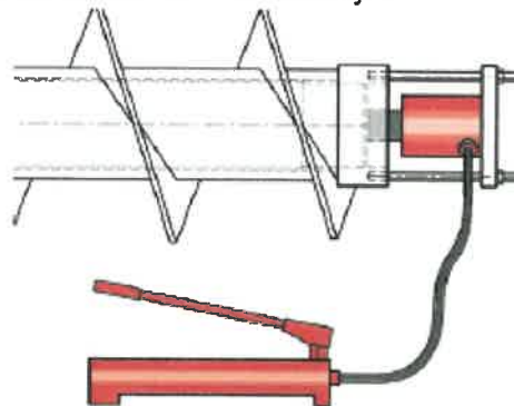
Rys. nr 6.13.28. Schemat wykonania opisanych czynności demontażowo- montażowych.
